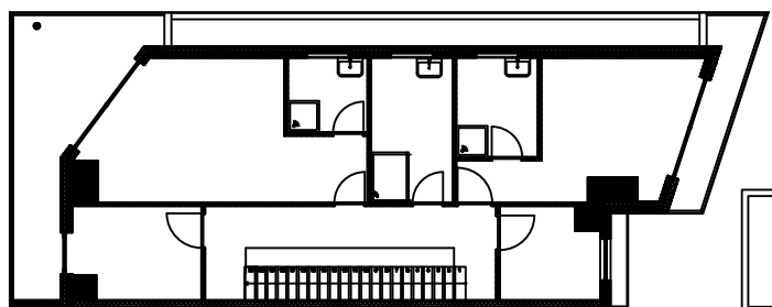
2 PLANTA ALTA VENTA4 1:200
