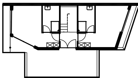
2 PLANTA ALTA VENTA2 1:200
